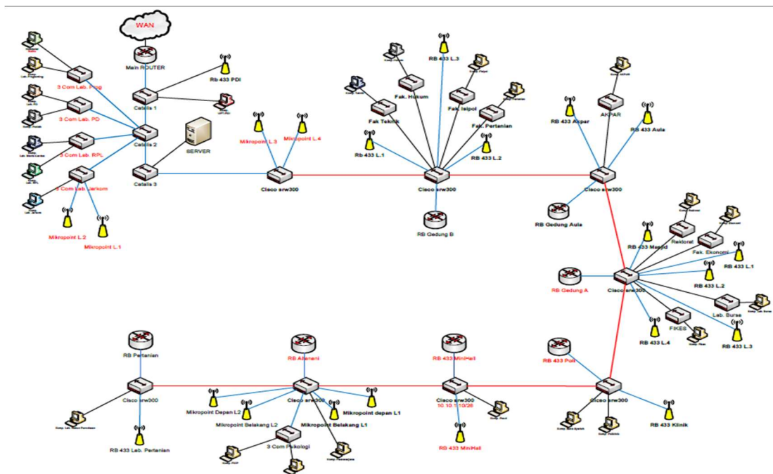
Gambar 1. Topologi yang akan dikonfigurasi menjadi WDS
