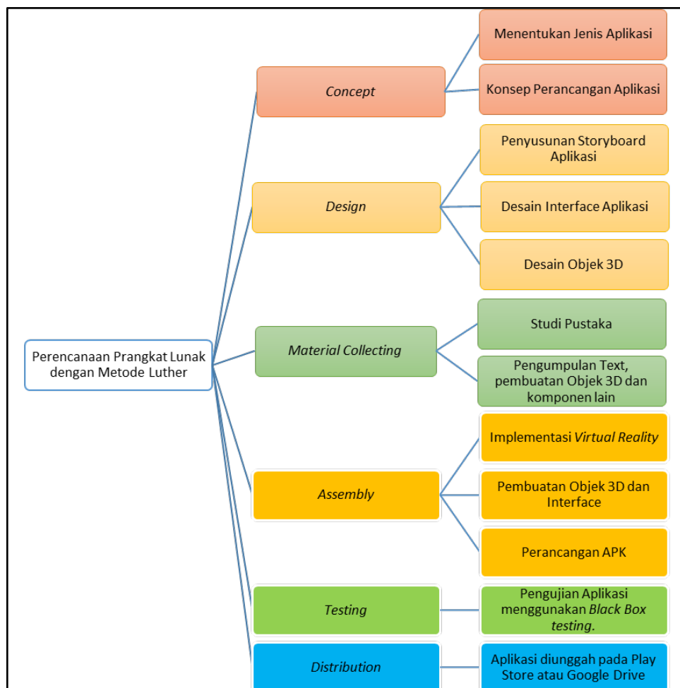
Gambar 2. Perencanaan Dalam Bentuk WBS
