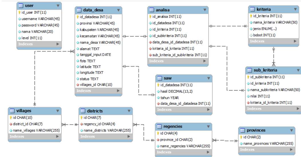
Gambar 3. ERD pada Sistem Bantuan MCK menggunakan SAW
